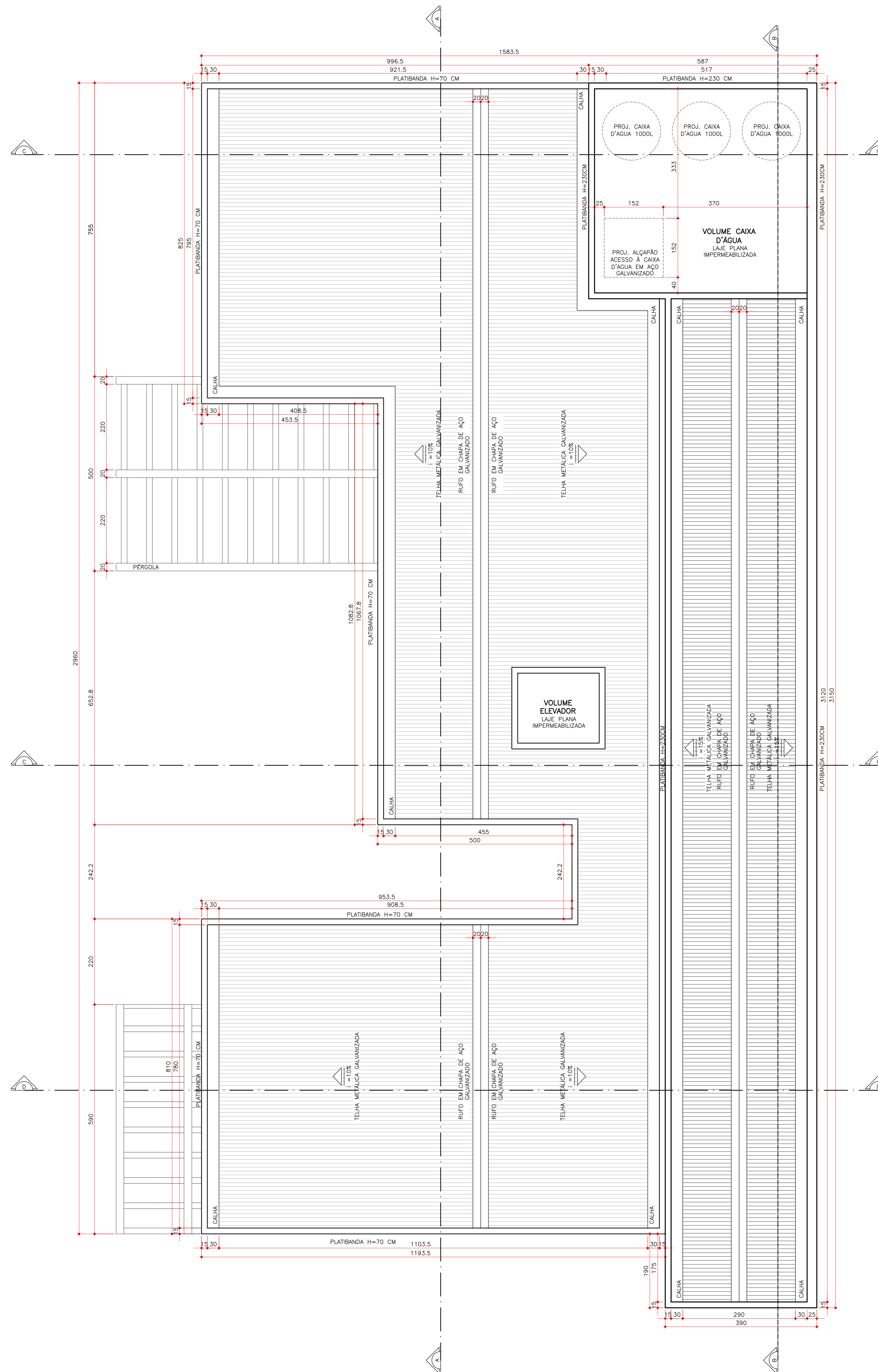
CENTRO ADM. SERRA AZUL DE MINAS PLANTA DE COBERTURA ESC 1/50
